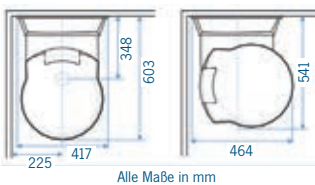
Draufsicht C 262 CWE/C 263 CS+CSL
