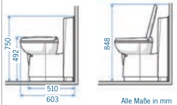
Seitenansicht C 262 CWE/C 263 CS
