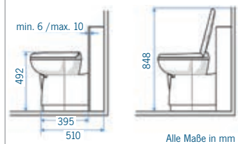
Seitenansicht C 263 S
