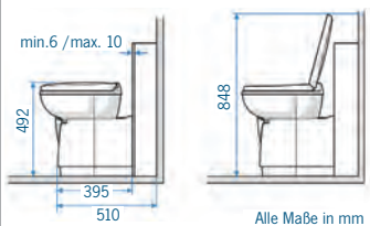
Seitenansicht C263 S
