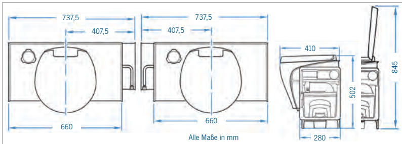
Fäkaltank 19,7 Liter
