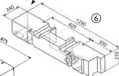
53 Liter EV 1104
