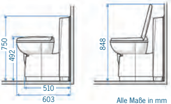
Seitenansicht C262 CWE / C263 CS
