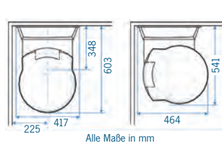
Draufsicht C262 CWE / C263 CS+CSL
